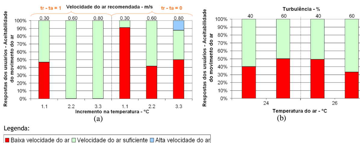
Figura 4 - Gráfico da aceitabilidade do movimento do ar tendo como referência as especificações da ASHRAE 55 (a) e ISO 7730 (b)
