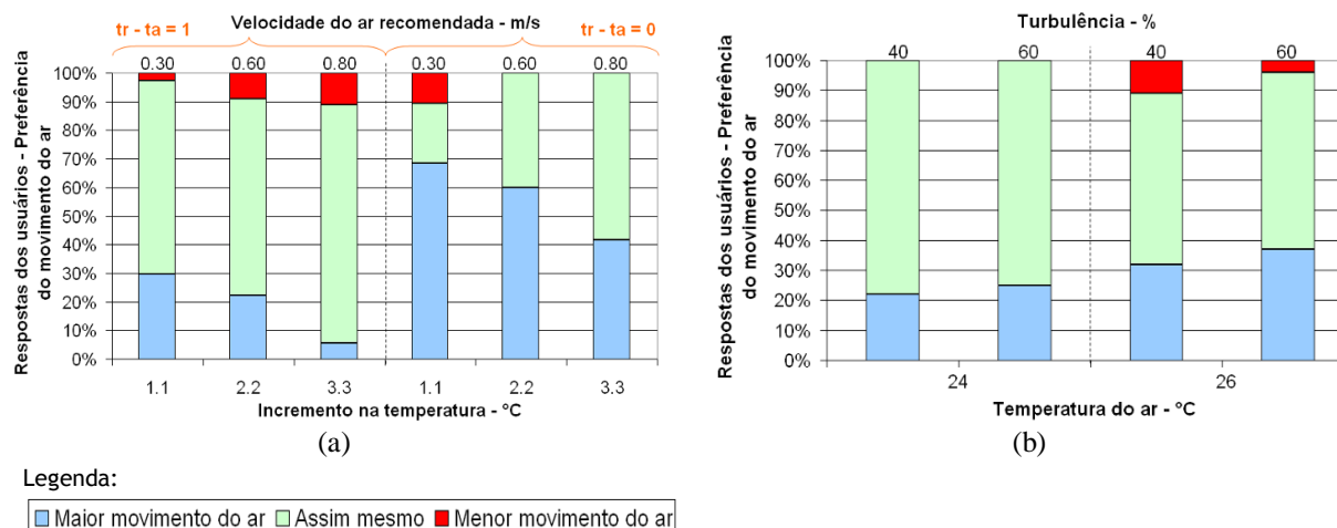
Figura 3 - Gráfico da preferência do movimento do ar tendo como referência as especificações da ASHRAE 55 (b) e ISO 7730 (a)
