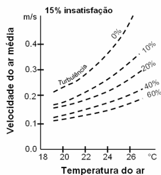
Figura 1 – Gráficos para determinação dos valores da velocidade do ar de acordo com a (A) ASHRAE 55 (2004) e (B) ISO 7730 (2005).
