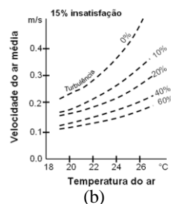
Figura 1 - Determinação dos valores da velocidade do ar de acordo com a (a) ASHRAE 55 (2004) e (b) ISO 7730 (2005), livremente adaptados e traduzidos dos originais
