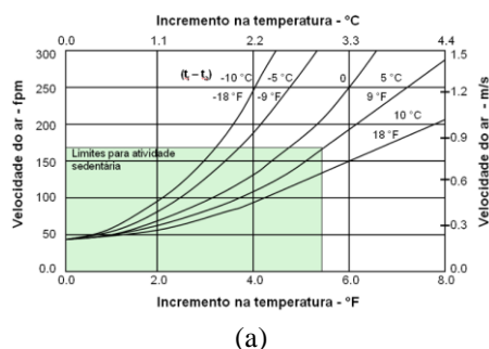
Figura 1 - Determinação dos valores da velocidade do ar de acordo com a (a) ASHRAE 55 (2004) e (b) ISO 7730 (2005), livremente adaptados e traduzidos dos originais
